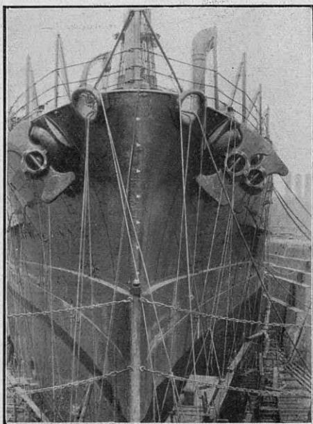
En Nueva York.—En dique seco, mostrando la coraza de la cintura del buque
