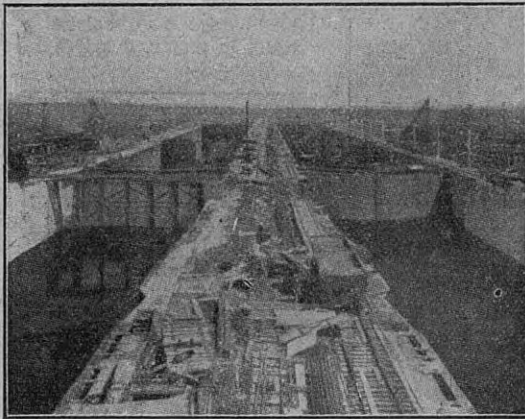
La disposición paralela de las esclusas. Ello permitirá a los navíos, yendo en sentido opuesto, franquear simultáneamente las esclusas y realizar una gran economía de tiempo al atravesar el canal
