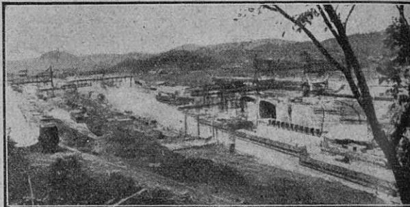
Una esclusa de Pedro Miguel, en vía de terminarse
