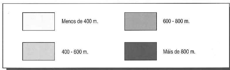
UNIDADES DE RELEVO E REDE HIDROGRÁFICA
