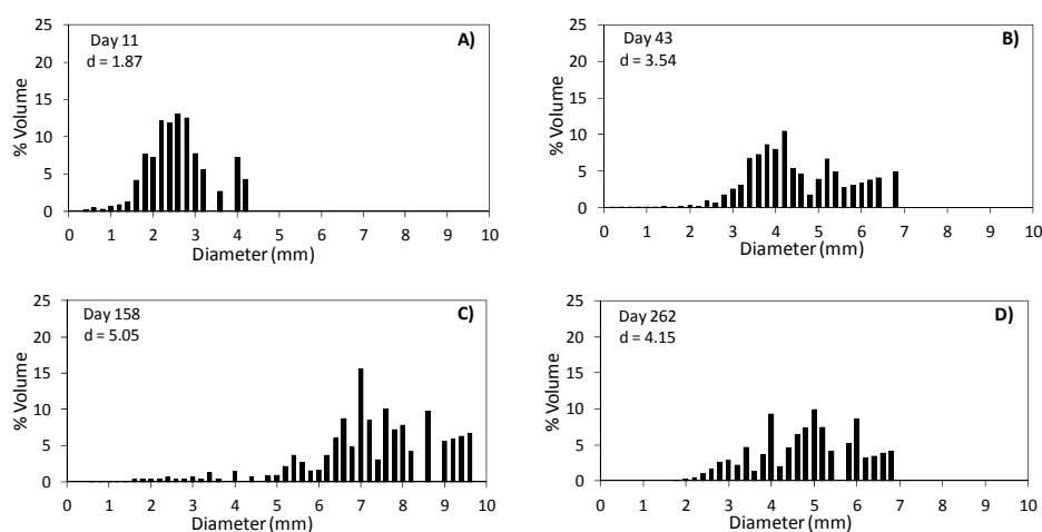
Figure 5.7. Volumetric size distribution (%). A) Day 11 (S. IA), B) day 43 (S. IA), c) day 158 (S. ID) and d) day 262 (S. II).
