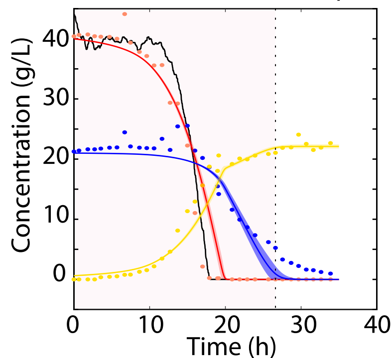
B.5. FERMENTATION 2 (26 h 45 min)
