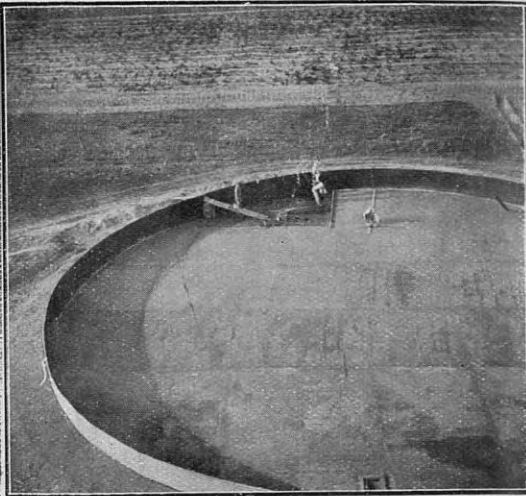
Colocando el piso a un tanque de 600.000 litros
