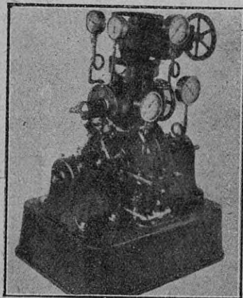
Turbina de alta presión de 200 caballos de potencia, en la instalación radienergética de Tesla
