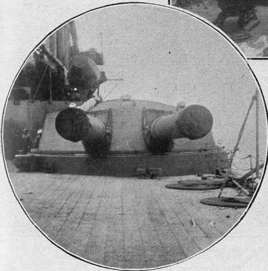
Una de las torres de las bandas (una por banda)
