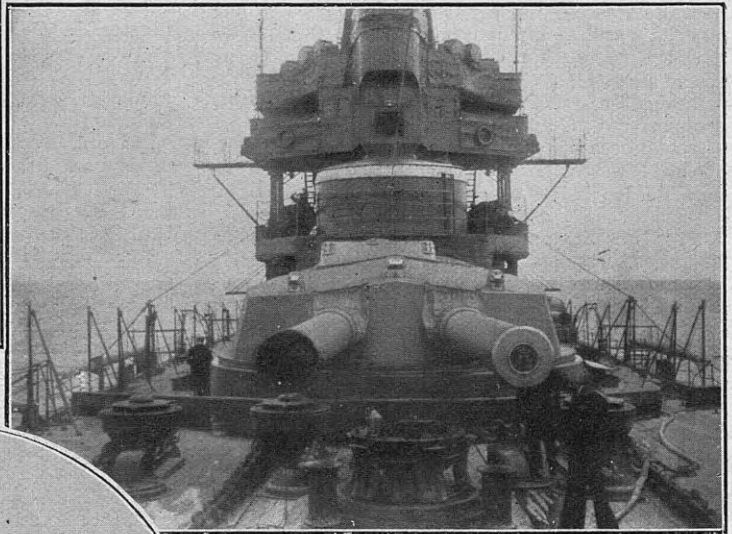
La torre de proa alojando sus dos respetables cañones de doce pulgadas
