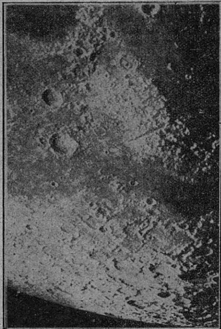
El Cáucaso, los Alpes y el Polo Norte de la Luna
