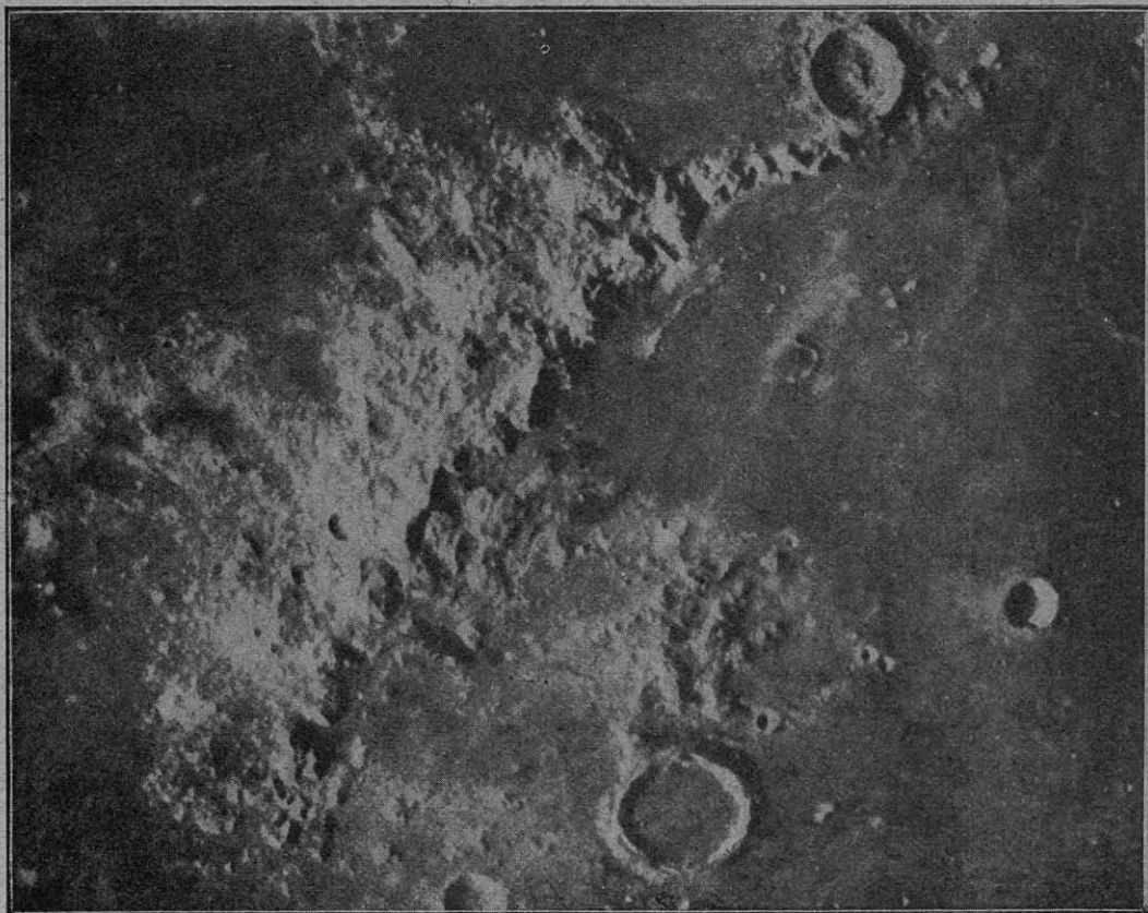
Los Apeninos lunares elevándose sobre las llanuras denominadas mar de los vapores y de la Putrefacción
