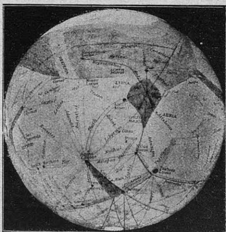
Mapa del planeta Marte
