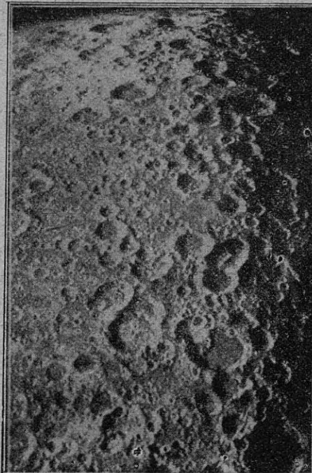
Una vista de la Antácluda lunar
