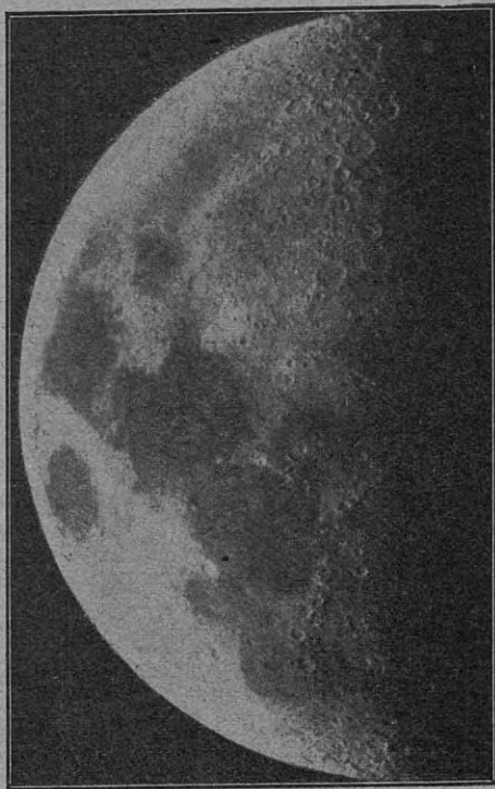
La Luna, vista a 3.000 kilómetros, con auxilio de la ecuatorial, del observatorio de París
