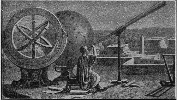
Hiparco, descubriendo una nueva estrella en Alejandría, cuyo descubrimiento le decidió a formar el primer catálogo de los astros
