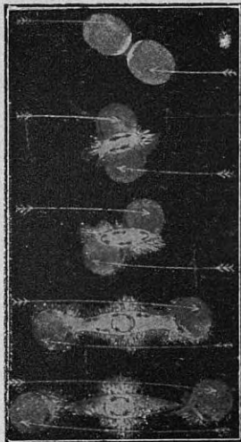
Las fases de la producción de una estrella nueva, según la teoría de Bickerton
