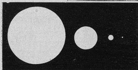
Tamaños relativos del disco solar visto, respectivamente, desde Mercurio, la Tierra, Júpiter y Neptuno
