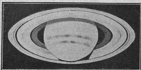
Saturno, con sus anillos, compuestos cada uno de millones de diminutos satelitoides
