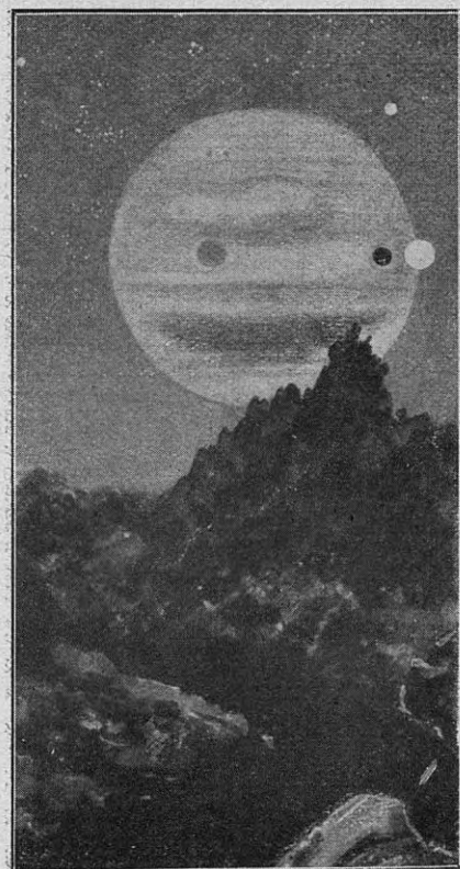
Júpiter y sus satélites interiores, vistos desde uno de los satélites más remotos del planeta gigante
