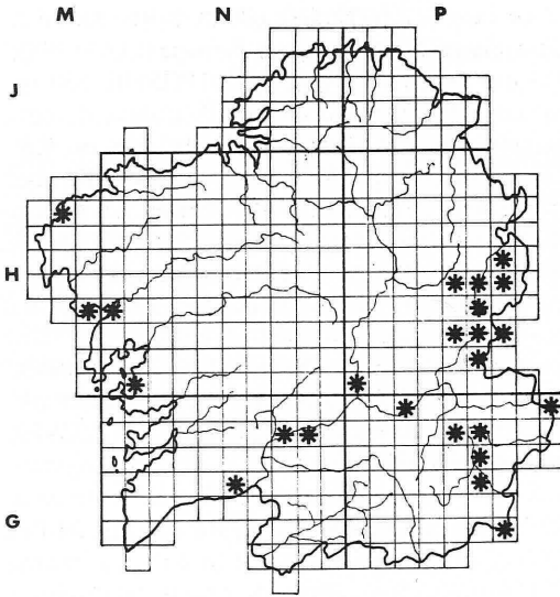
Fig. 1. Distribución de Arabis juressi Rothm. en Galicia.
