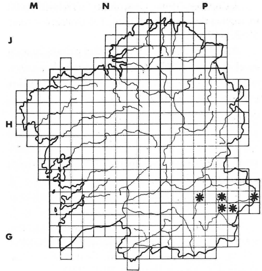
Fig. 2. Distribución de Arabis stenocarpa Boiss. & Reuter en Galicia.
