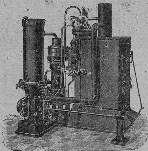
Vista de una instalación completa ECONÓMICA, con desnatadora "BALTIC" a turbina, para 1.000 litros por hora
