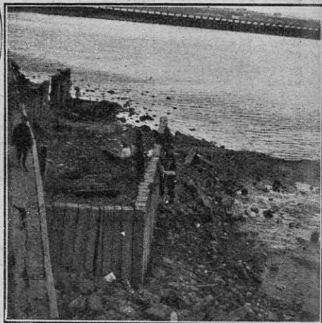
Quedó en seco la parte del murallón exterior del puerto, obra de defensa que corre paralela a la línea de diques y dársenas
