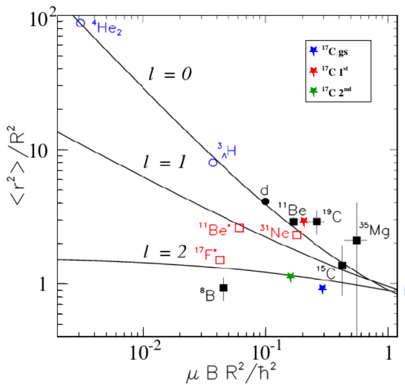
Figure D.5: Lei de escala adimensional definida por K. Rüssager para halos de dous corpos. O puntos negro representa o deuteron, círculos azuis e cadrados vermellos baleiros indican modelizacións e cálculos teóricos, mentres cadrados negros baleiros son deducidos de datos experimentais. As estrelas azul, vermella e verde representan o estado fundamental e o primeiro e segundo estado excitado no {}^{17}\text{C} (Adaptada de [91])
