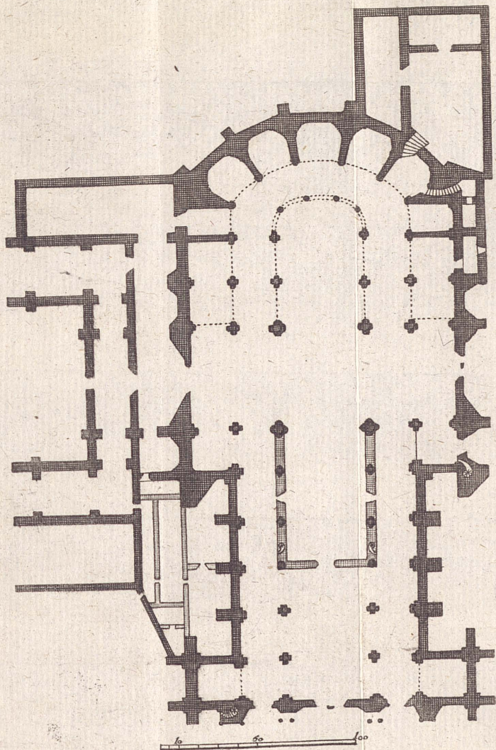
Planta de la Catedral de Leon.
