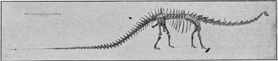
Restauración del Diplodocus según Marsh y cómo se exhibe en el Museo de La Plata
