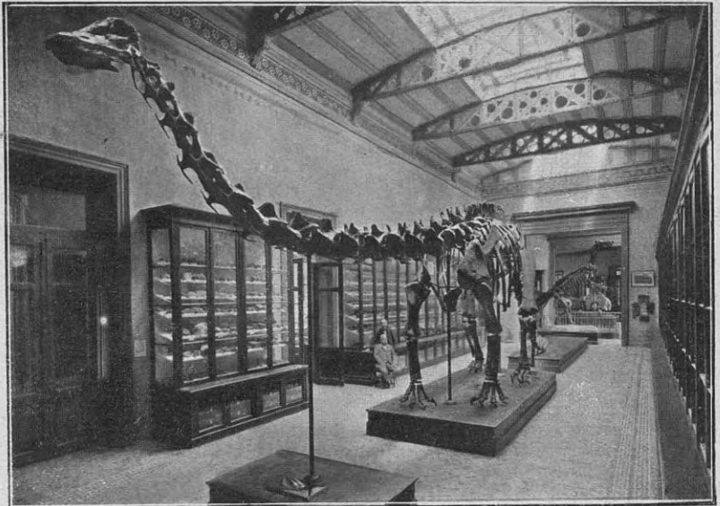
El Diplodocus Carnegii en el Museo de La Plata
