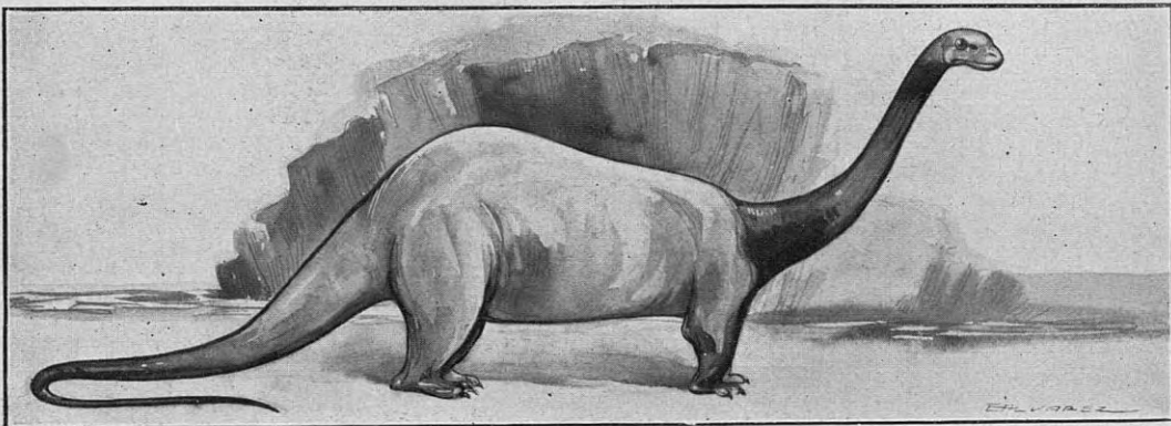
Reconstrucción ideal del Diplodocus según Pullenberg, y que pronto ha de colocarse en el bosque de La Plata
