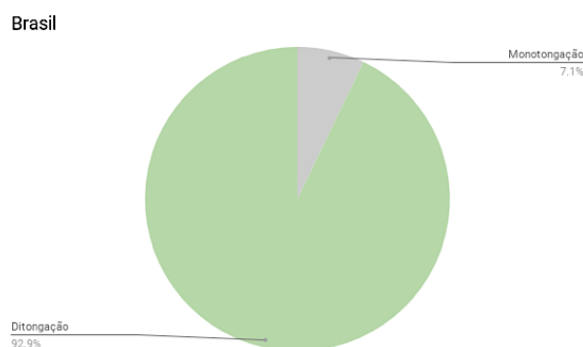
Gráfico 1: distribuição da monotongação e ditongação por parte dos falantes brasileiros. Elaboração própria a partir de dados do dicionário Forvo .
