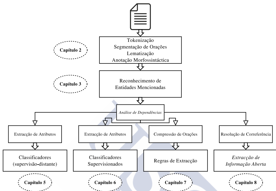
Figura 1.2: Diagrama dos processos realizados em cada capítulo. A entrada (acima) é texto plano, sendo avaliadas quatro estratégias de extracção de informação (abaixo) nos Capítulos 5 a 8. Os elementos em itálico não foram realizados especificamente nesta tese.
