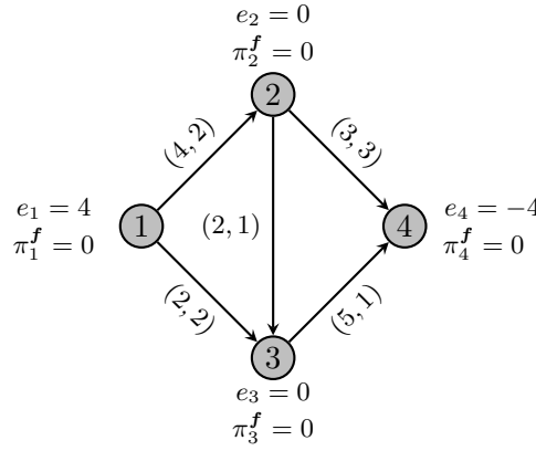
Figura 2.9: Ejemplo de PFCM. Red R^f en la iteración I.
