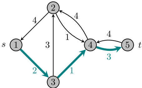
(c) C^f encontrado con el algoritmo de etiquetado.
