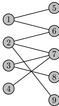
Figura 4.2: Ejemplo de problema de emparejamiento bipartito de máxima cardinalidad.
