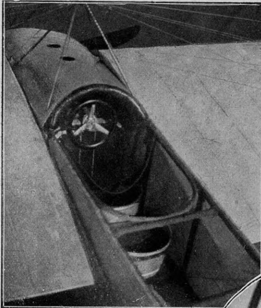
Los asientos del piloto y del pasajero, y el volante de dirección, con sus correspondientes cables, en un monoplano de tipo Castaibert, aparato cuya sencillez de manejo facilita el aprendizaje
