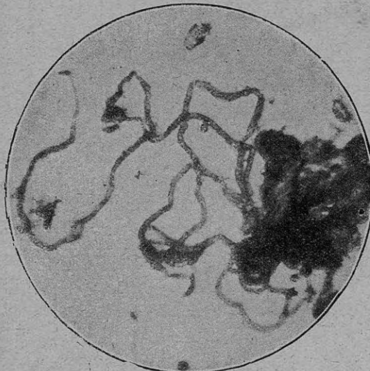
Germinación aparente de la cineonina en el ácido fosfomolibdico.
