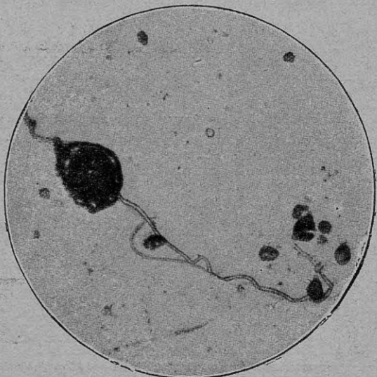
Célula artificial de estriquinina y ácido fosfo-túngstico
