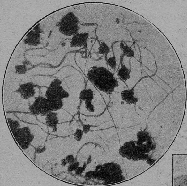
Germinación aparente de las anilinas
