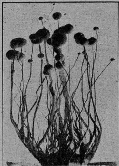
Crecimientos osmóticos obtenidos por el profesor Stephane Leduc, de Nantes
