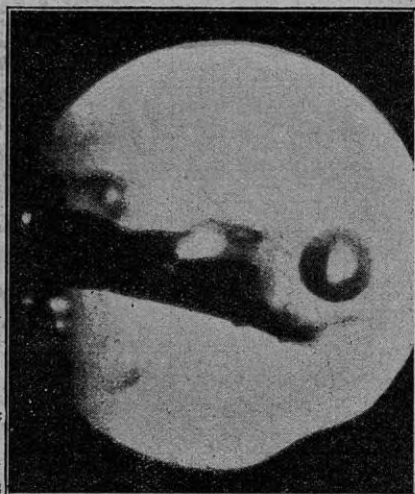
Circulación activa de burbujas de oxígeno
