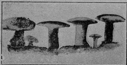
Hongos minerales obtenidos por Butcher
