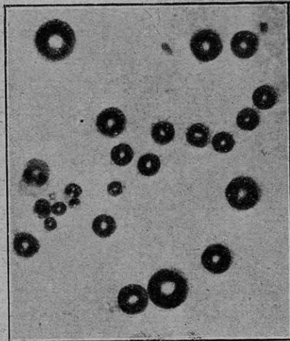
Descomposición del agua oxigenada
