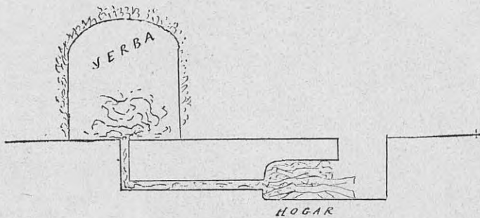
Esquema de barbacuá
