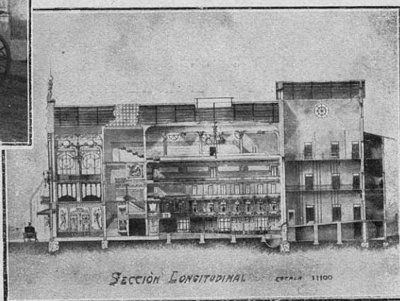
Sección longitudinal, con la sala para 1.400 personas
