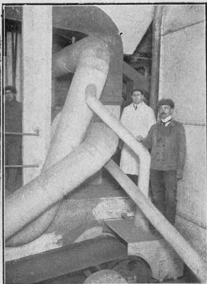
Cinta conductora de trigo y caños aspiradores de polvo
