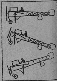
Demostración de cómo el centro de presión (marcado por la flecha) cambia de sitio en un monoplano del tipo corriente
