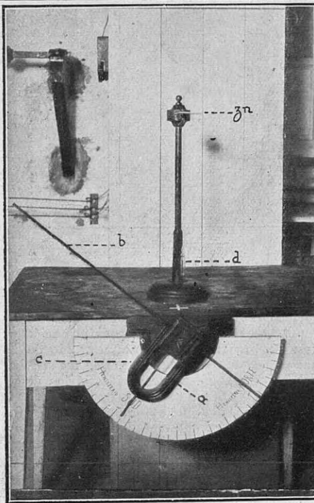
El magnetoscopio Ducco: a, imán cuyo fin es proporcionar una barra imantada sin puntos consecuentes; b, barra de hierro que suple al eje magnético de la Tierra; c, cuadrante que indica las desviaciones de la barra, acusando las distintas latitudes terrestres; d, nivelador para determinar el centro en las experiencias; zn, placa de zinc sobre la cual se coloca el cuerpo cuya influencia quiere estudiarse. (El zinc calentado a 100° pierde toda su influencia por un período de 24 horas)
