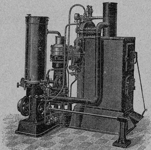
Una cremería con desnatadora "BALTIC" desde 1.000 a 4.000 litros por hora
