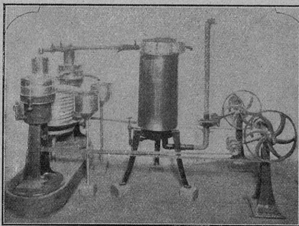
Vista de una instalación completa ECONÓMICA, con desnatadora "BALTIC" a turbina, para 1.000 litros por hora
