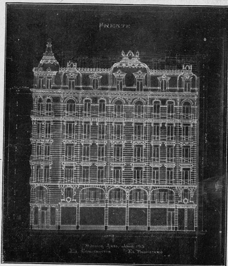
Plano del gran edificio que el señor Carlos Rasetti está haciendo construir en el mismo terreno donde estaba la casa de Salomón
