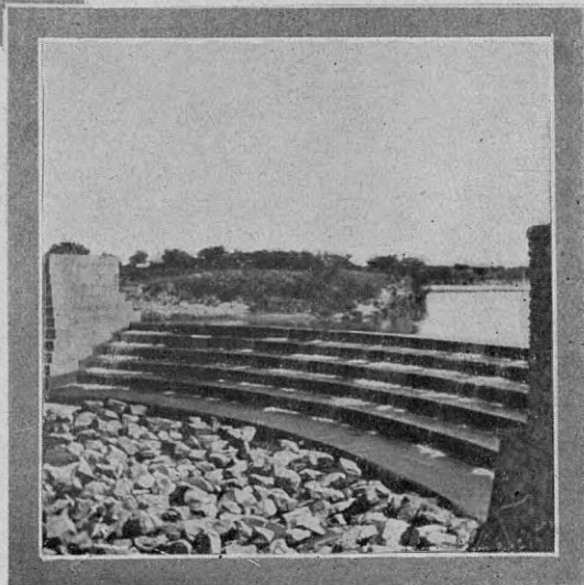
Dique nivelador de Mercedes, en el río Quinto
