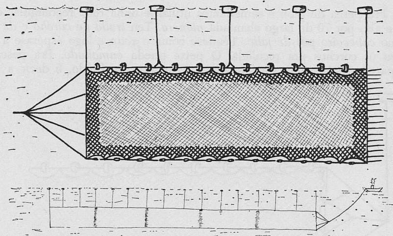
Fig. 12: xeito
