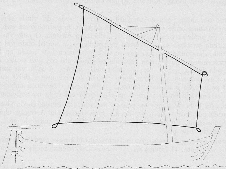
Fig. 5: vela
