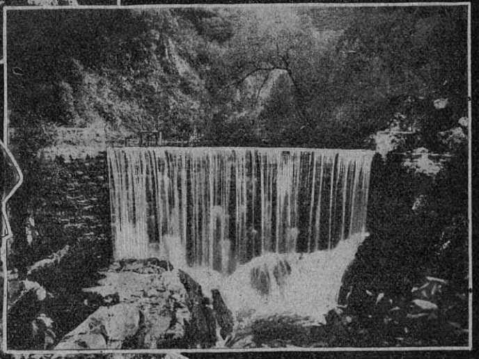
Valle Hermoso. — Dique Marcuzzi rebalsando. Esta represa contiene muchos miles de metros cúbicos de agua purísima de vertientes
