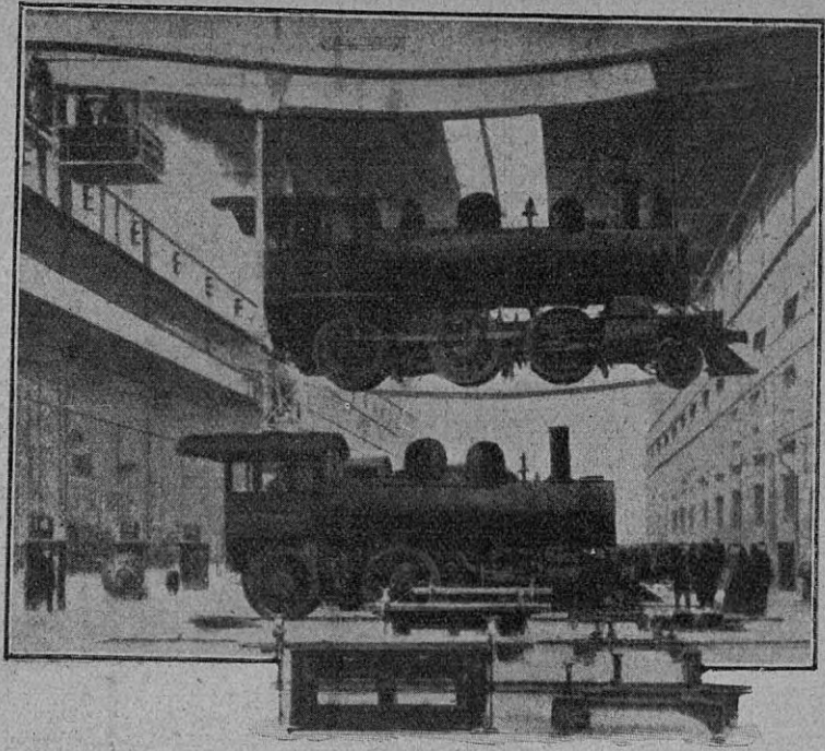
Esta fotografía está tomada en el momento de levantar una locomotora de 80 toneladas
