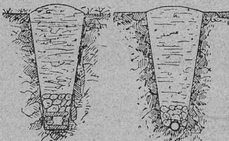
Drenaje con piedras y canal interior
