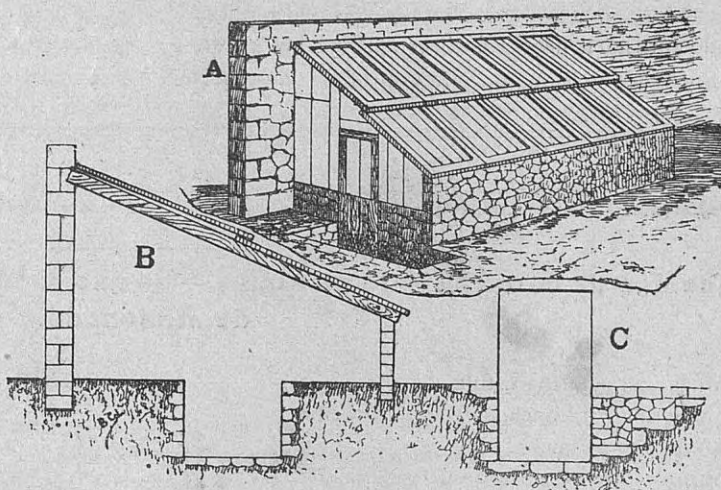
Estufa: A perspectiva; B corte transversal; C puerta, mostrando la situación de la escalera
