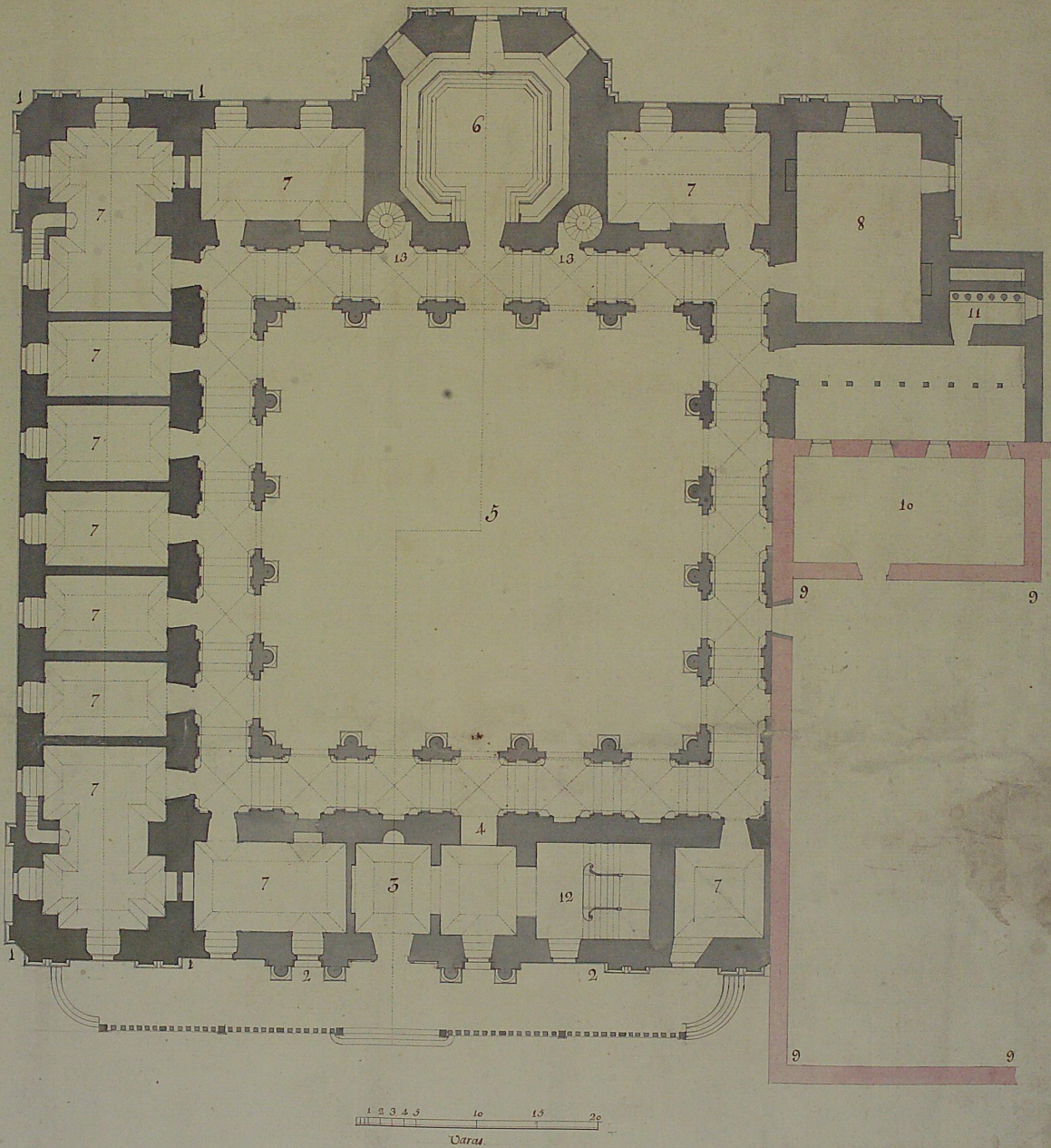
Plano I. que representa la Ychnographia, ò vestigio Horizontal de toda la Obra de la Universidad correspondiente al terreno
