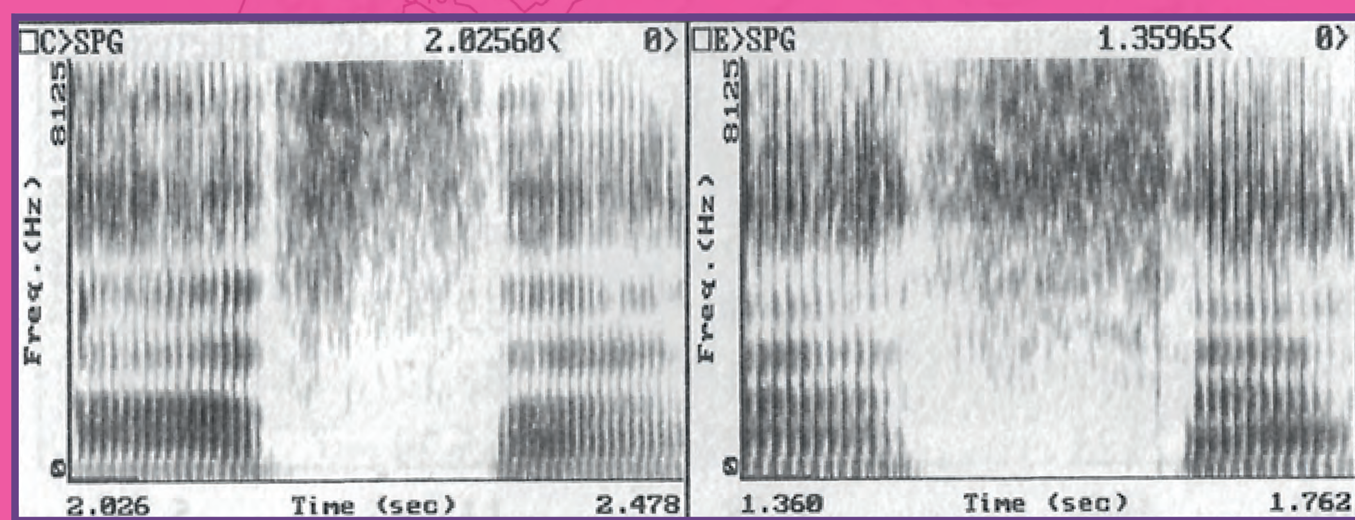
Figura 1. Espectrogramas das fricativas [f] e [θ]
