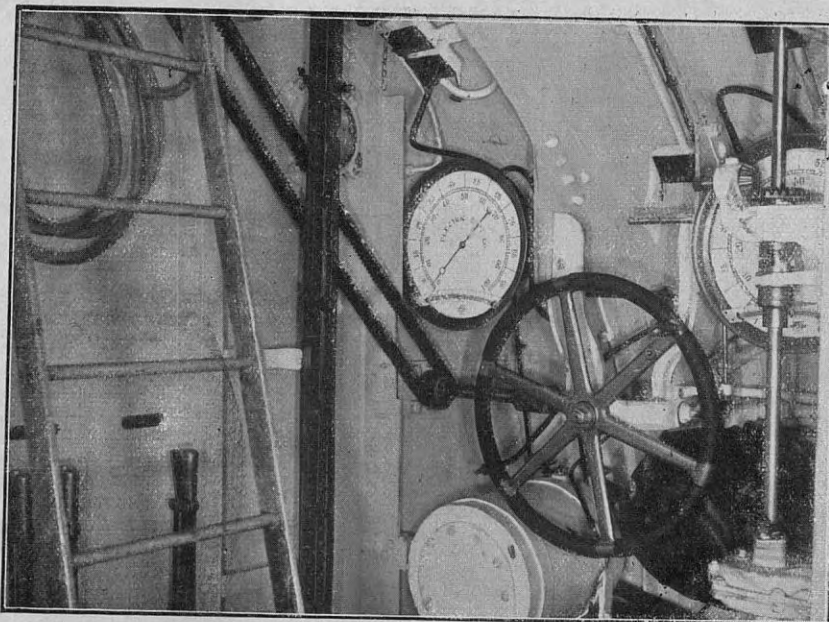
Volantes para la sumersión. (Las esferas graduadas son los registradores de profundidad)
