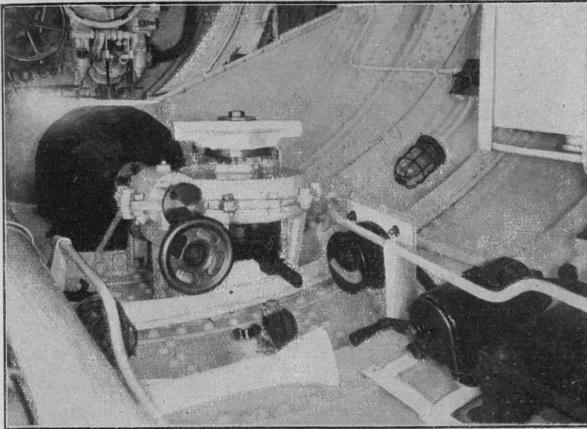
El cabrestante del ancla, que funciona por medio de un motor eléctrico y está rigidamente unido al techo, ó sea, á la cara interior de la cubierta del submarino
