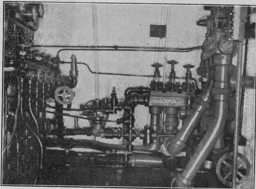
Válvulas de aire, para inundación de los estanques de sumersión
