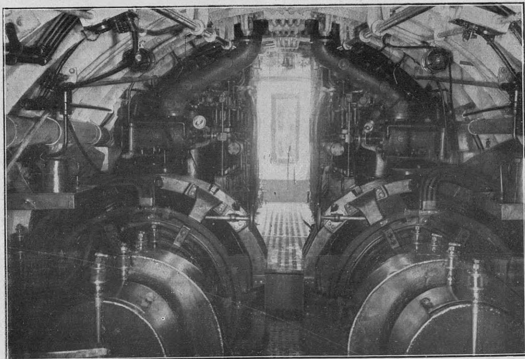
Cámara de los motores principales. (En primer plano y a ambos lados, se notan los eléctricos, y hacia el fondo los de combustión interna, para navegar debajo y en la superficie del agua, respectivamente)
