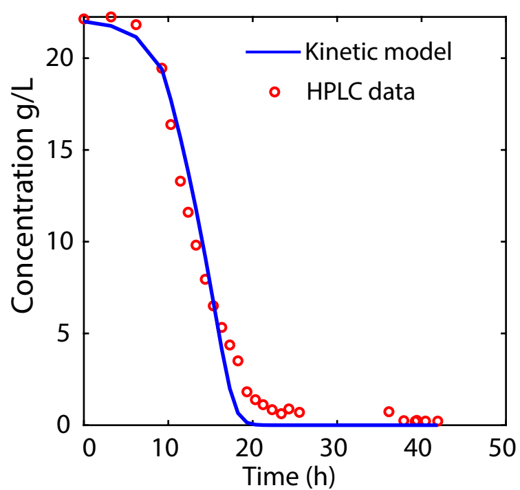
B. XYLOSE
