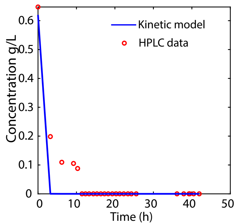
D. FURFURAL
