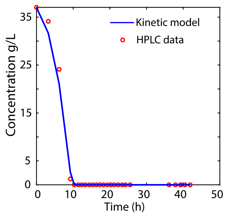
A. GLUCOSE
