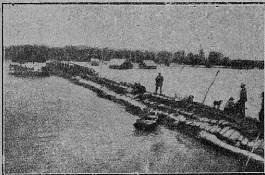
Reparación provisional de un dique con sacos de tierra durante la crecida
