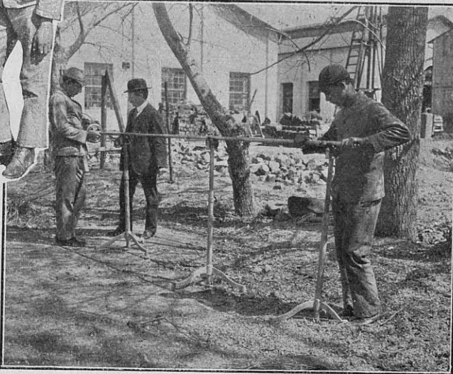
Calibrando un cañón A. T. R. de 12 con el hipocelómetro (estrella móvil). — Con este instrumento se pueden apreciar con toda facilidad diferencias de un centésimo de milímetro
