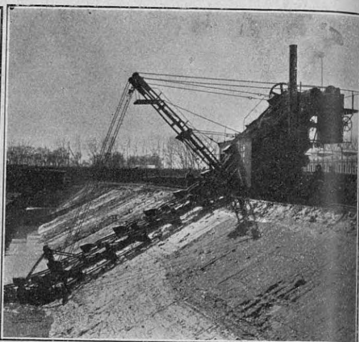
Una de las excavadoras mecánicas de la empresa Bonneu, Ibero, Parodi y Figini, empleadas en las obras de los nuevos depósitos
