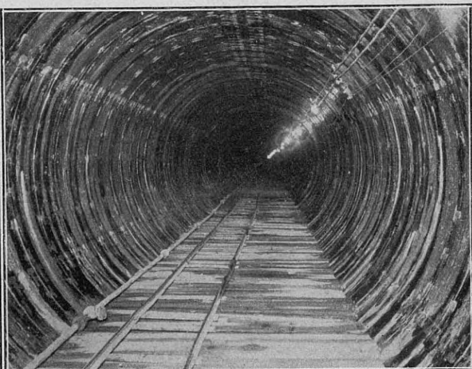
Vista interior del gran túnel de toma que fué visitado por la comitiva
