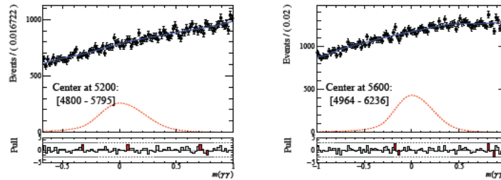
Figura C.5.6: Dous dos axustes realizados a unha potencial sinal e a un fondo combinatorio.
