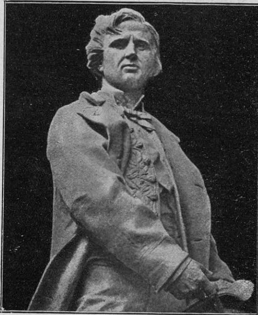
Urbano Leverrier, cuyo descubrimiento de Neptuno fué una de las más brillantes confirmaciones de la ley de la gravitación
