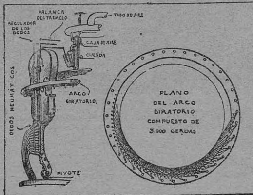
Detalles del mecanismo del violín
