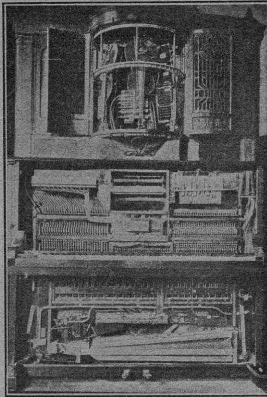
El violín mecánico, combinado con piano
