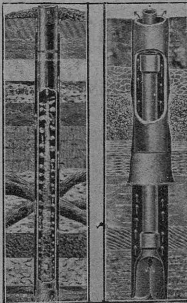
Zapata giratoria y perforadora hidráulica
