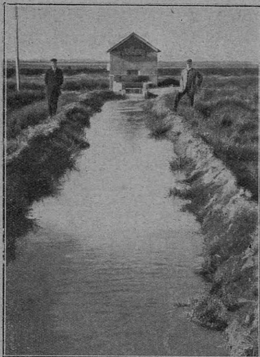
Instalación que comprende una bomba centrífuga de 20 centímetros, impulsada por un motor de 30 caballos, la cual eleva 2.200 galones por minuto a una altura de 28 pies
