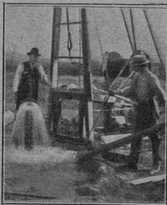
Concluyendo de perforar un pozo artesiano
