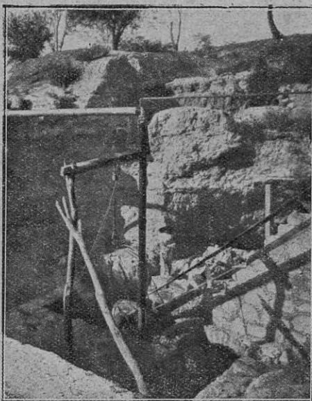
Construyendo una presa en una hacienda mejicana. Bomba centrífuga impulsada por correa
