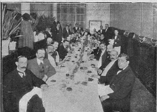
Durante el banquete ofrecido el 18 al juez de paz de la sección 16.ª, señor F. Oteguí
