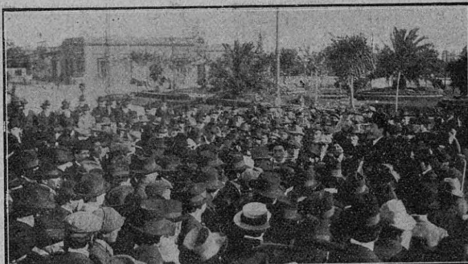
En La Plata.—El ciudadano Alejandro Mantecón proclamando la candidatura del doctor Alfredo L. Palacios para gobernador de la provincia de Buenos Aires, en la plaza Italia
