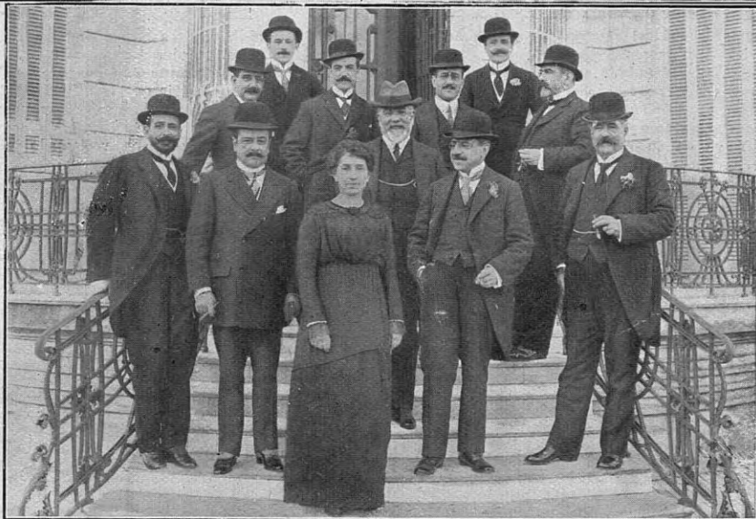
El ministro de España, la señora de Calzada, los doctores Rafael, Fermín y César Calzada, Avellaneda, Luis Méndez Calzada, Ortiz y San Pelayo
