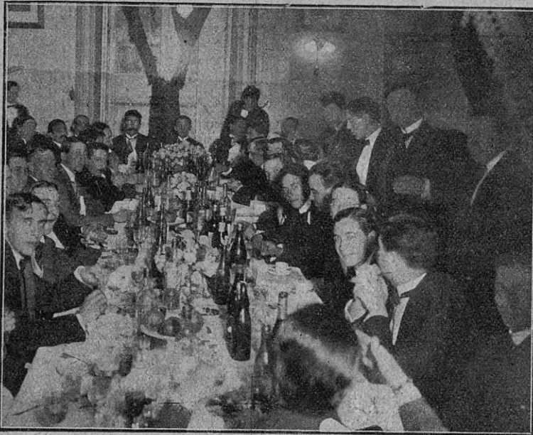
En Mendoza, los amigos del señor David Guinazú le despidieron de la vida de soltero con una comida, con motivo de su enlace con la señorita María Elcira González
