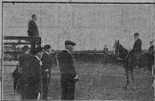
El director del movimiento unionista sir Edward Carson arengando a los voluntarios de Belfast
