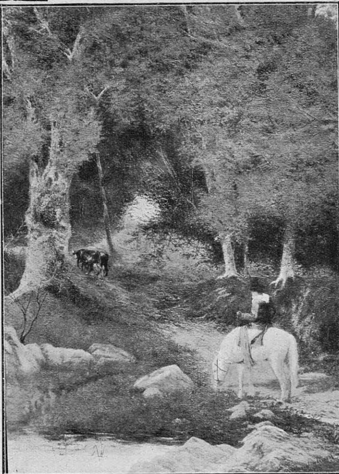
“Internándose en el bosque”. Paisaje en la quebrada de Lules
