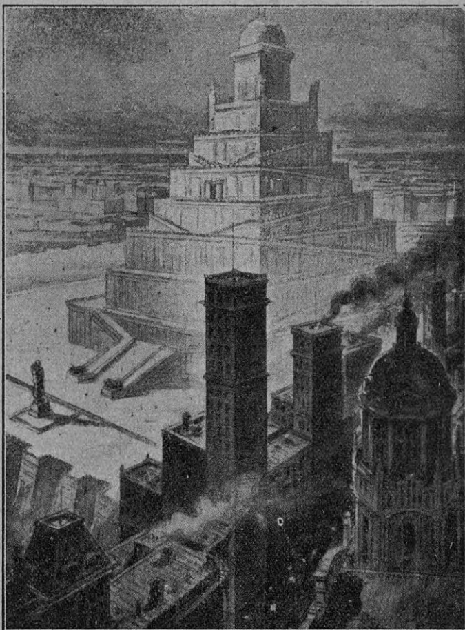
La antigüedad y los Estados Unidos. Los modernos rasca-cielos son aun pequeños comparándolos con los 200 metros de altura de las tumbas de los reyes de la Caldea, tal como la de Nabuccodonosor
