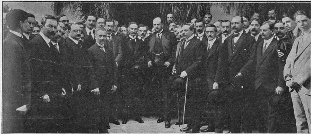
El doctor Beláustegui y el intendente Anchorena, con motivo de la toma de posesión por el primero, del cargo de Director de la Asistencia Pública
