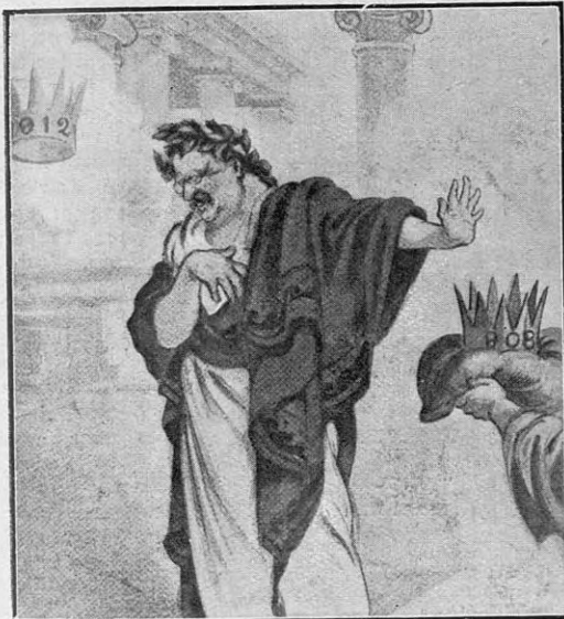
Roosevelt rechazando pudorosamente el título de César. (Del Puck)
