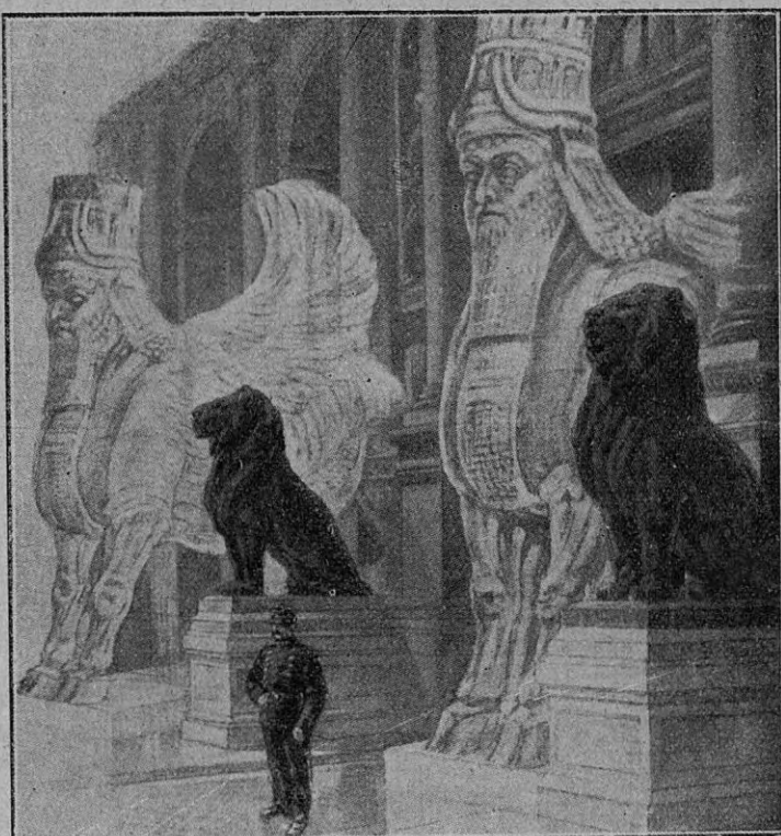
Toros antiguos y leones modernos. Gigantescos toros alados que miden seis metros de alto, comparados con ellos son minúsculos los dos grandes leones que flanquean la entrada del "Hotel de Ville" de París
