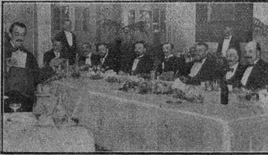
El popular poeta madrileño Antonio Casero leyendo una poesía en el banquete dedicado al señor Francos Rodríguez
