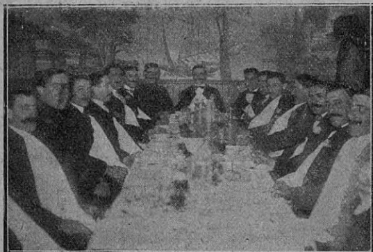
En atención al reciente ascenso policial del señor Amadeo Moroni, sus amigos le ofrecen una comida
