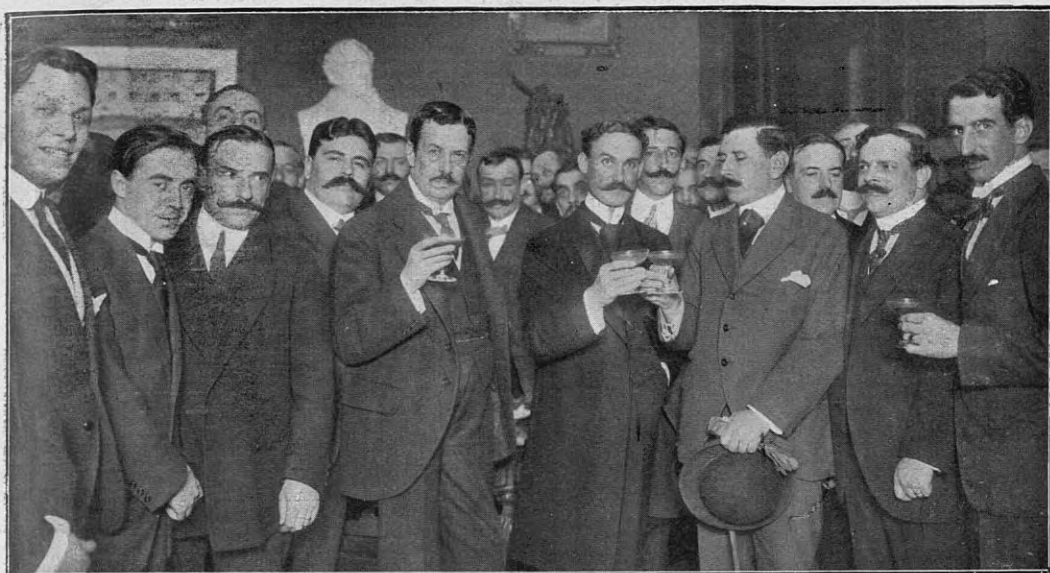
En la Municipalidad, bebiendo una copa de champagne, con motivo de la reelección del intendente, doctor Joaquín S. de Anchorena
