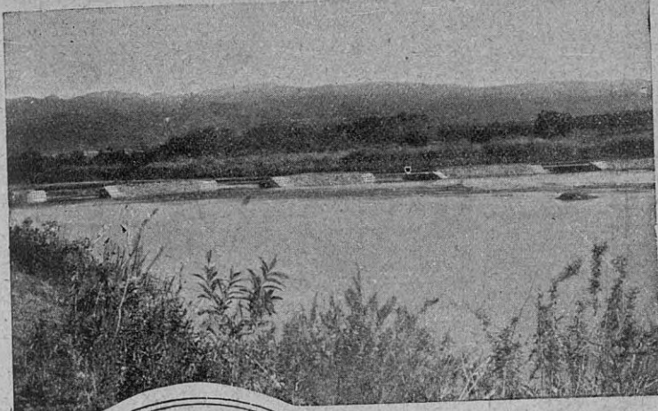
Puente mandado construir por el propietario de los terrenos que se venden, exclusivamente para el servicio del pueblo y balneario Anizacate.
