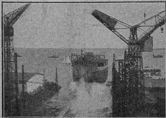
Botadura del acorazado francés "Lorraine", en Saint-Nazaire
