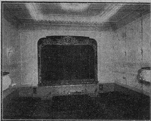
Vista parcial de la sala, tomada desde el fondo
