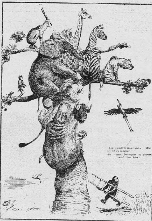
Medidas de precaución tomadas por las fieras africanas cuando supieron que Roosevelt estaba en el Cairo. — Las fieras: "¡Chist! Miren que ya viene". (Caricatura de Homer Davenport en The Evening Mail , de Nueva York)
