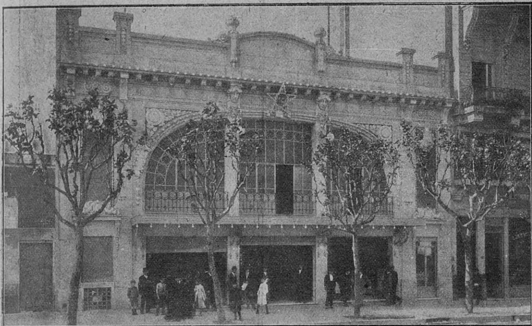
Vista exterior del lujoso cinematógrafo inaugurado recientemente en la calle Corrientes 2750-73
