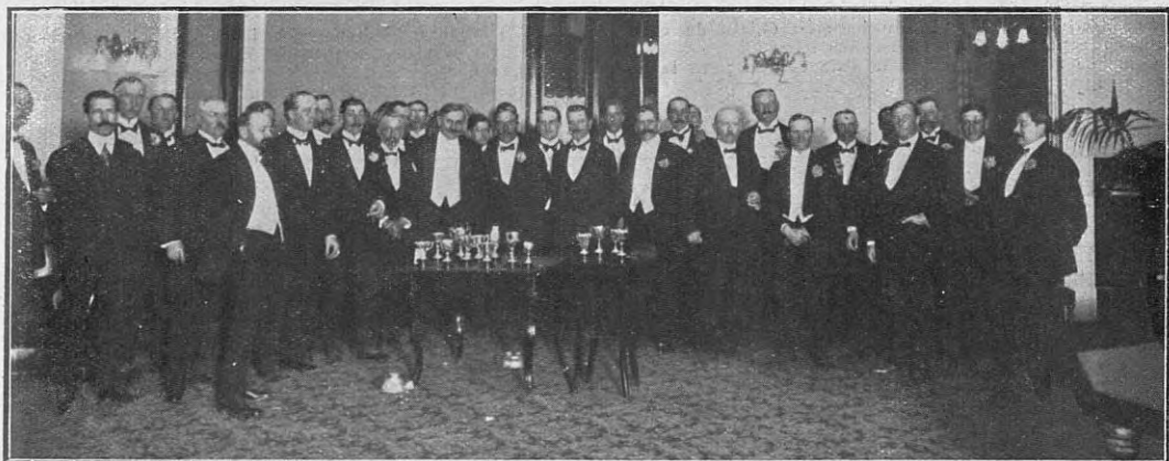
El 21 por la noche, durante la distribución de las copas correspondientes a este torneo, en el Club Social
