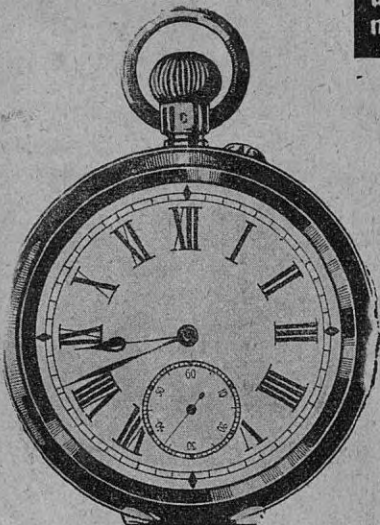
Premio núm. 9.—Un reloj de oro 18 kilates para caballero. Valor pesos 120.
