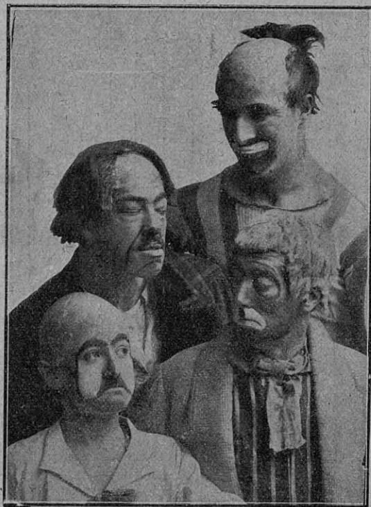
Los Rilo, acróbatas saltarines excéntricos
