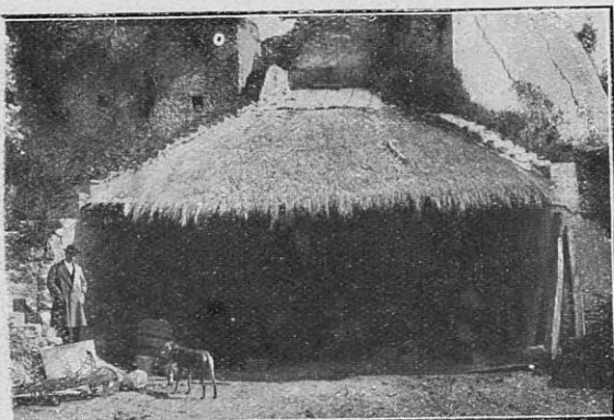
Horno sistema criollo
