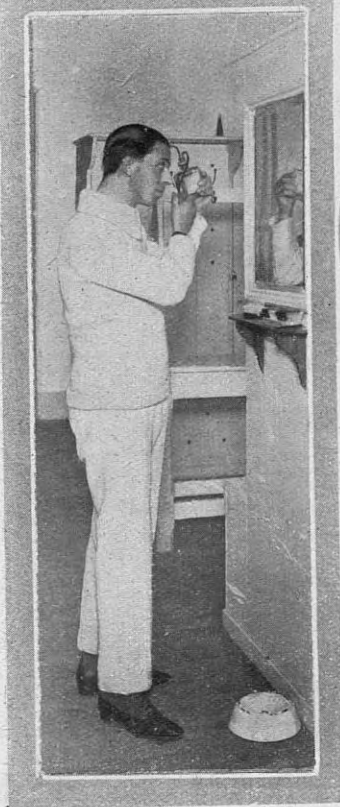
En el "toilette" del "R. C. A".—A. L. Graf, pulverizándose
