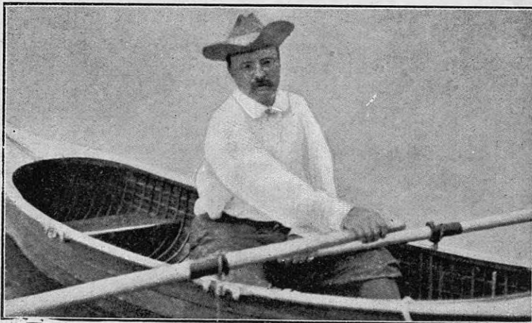
El remo es uno de los ejercicios favoritos de Roosevelt
