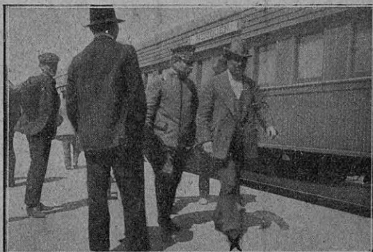
El jefe policial de Río Negro, señor Hector Moffard, recorriendo las poblaciones de su territorio.—A su llegada a Colorado
