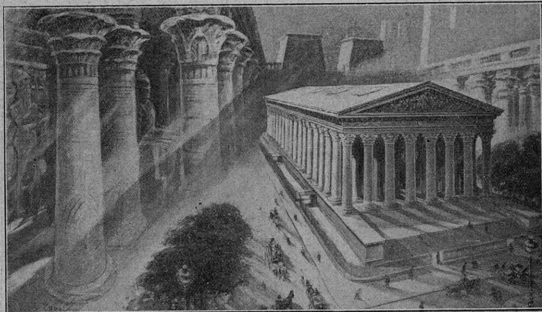
Sueño y realidad. La superficie de Karnak en Louksor es de 102 metros por 51 o sean 5202 metros cuadrados. El Louvre mide 118 metros de costado, 134 columnas rodean a Karnak, las de el ala central son del grueso de la columna de Vendôme y sostienen un plaón de una terraza de piedra de 23 metros de altura
