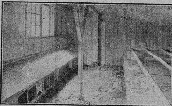
Un buen modelo de dormitorio para aves
