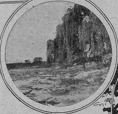
En las orillas del Anizacate
