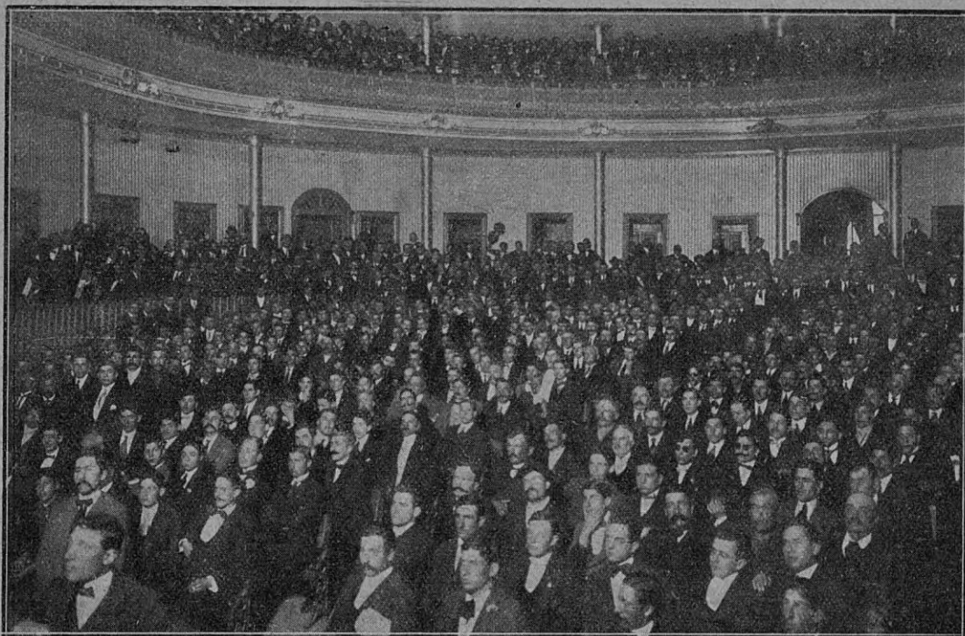
Aspecto del teatro Olimpo, durante la proclamación de la fórmula socialista "Alfredo L. Palacios-Alfredo J. Torcelli", candidatos a la futura gobernación y vice de la provincia de Buenos Aires, el domingo último, con asistencia de 3.000 ciudadanos
