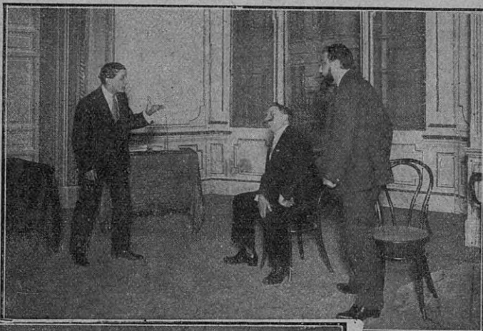
Pablo Podestá, Escarcela y Alippi en una escena del segundo acto
