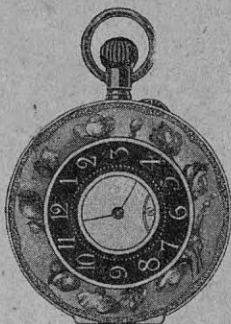
Premios núms. 12 y 13.—Dos pendientes con brillantes, perlas y esmalte en el anverso y un reloj en el reverso. Valor $ 85 c/u.
