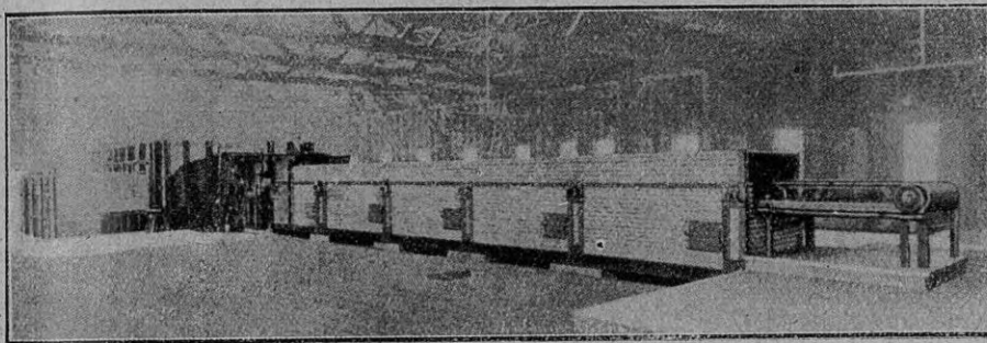
Vista completa de los hornos con la mesa de cortar las planchas de vidrio
