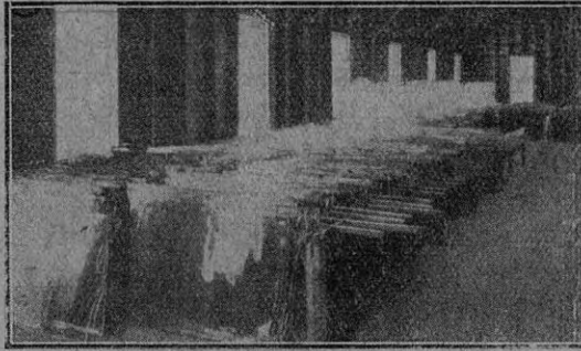
Planchas de vidrio obtenidas por el procedimiento mecánico de Colburn
