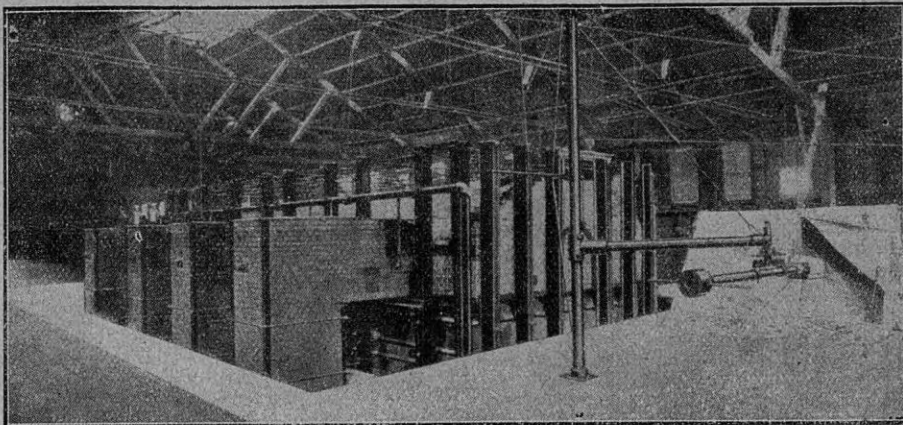
Depósito de la pasta de vidrio fundido con el mecanismo de carga
