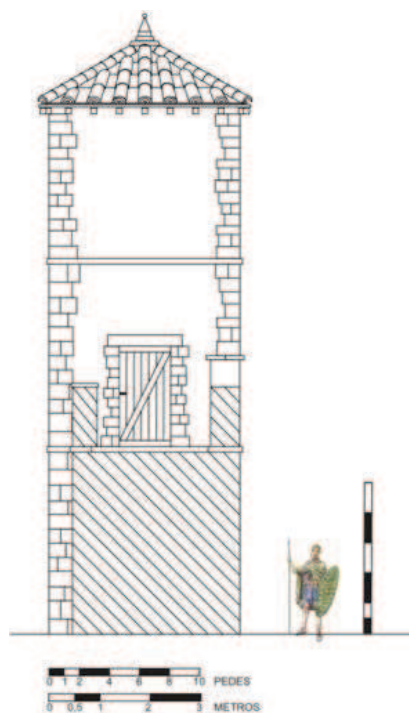
Figura 3.- Torre de intervalo. Hipótesis reconstructiva.
