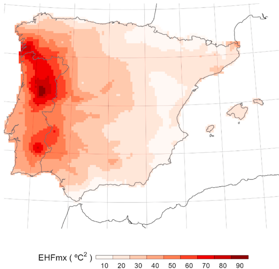
Fig. 11. Maximum EHF for the period 2018-07-29 to 2018-08-09 (in ^{\circ}\text{C}^2 ).
