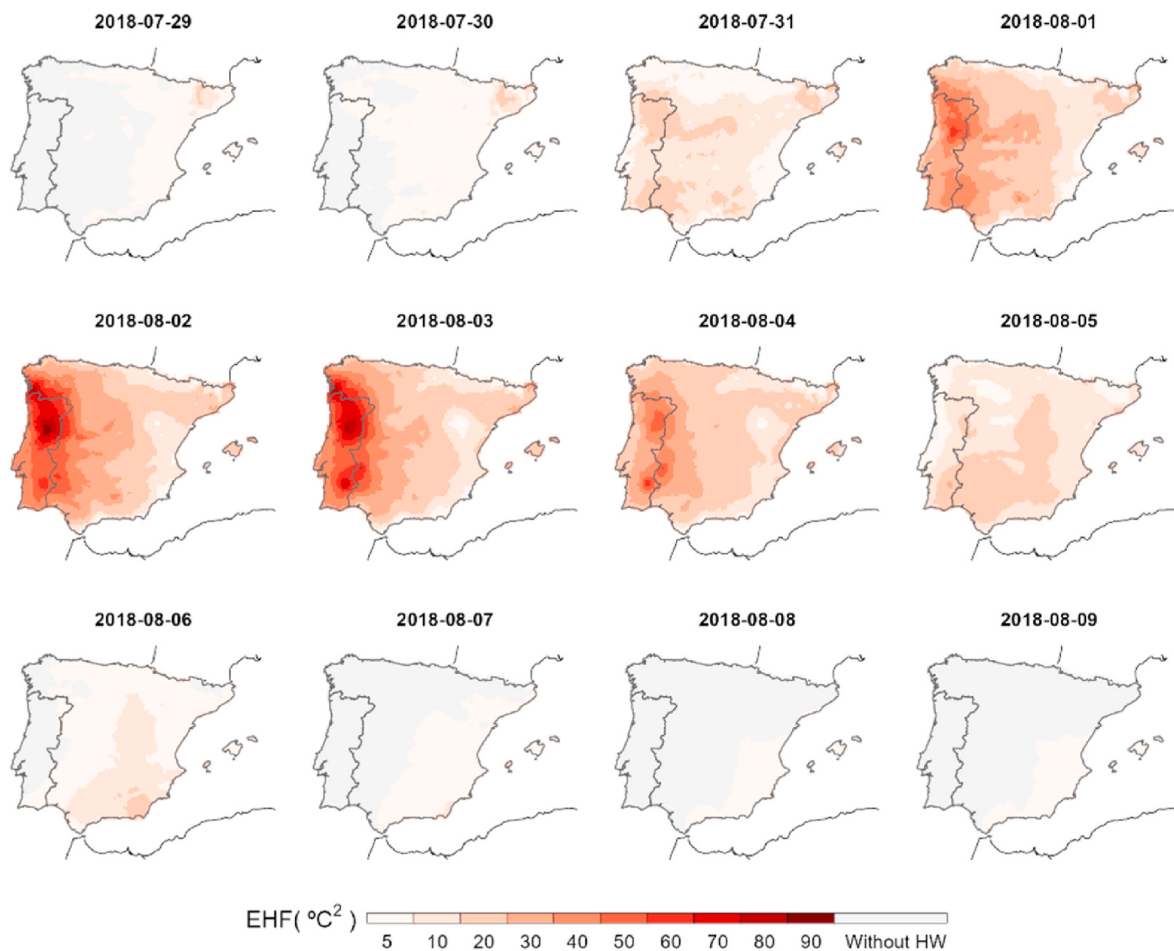
Fig. 10. EHF index values for the period 2018-07-29 to 2018-08-09 (in ^{\circ}\text{C}^2 ).
