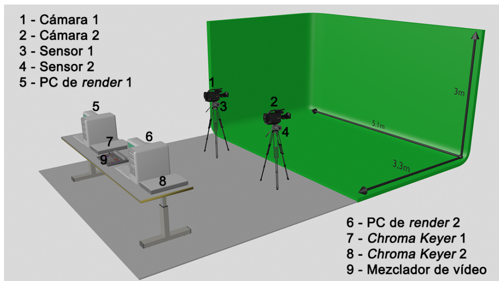
Figura 3.1: Diseño del plató virtual de televisión de la Facultad de Ciencias de la Comunicación de la Universidad de Santiago de Compostela
