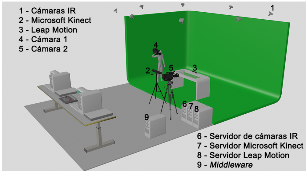
Figura 4.19: Configuración final del plató
