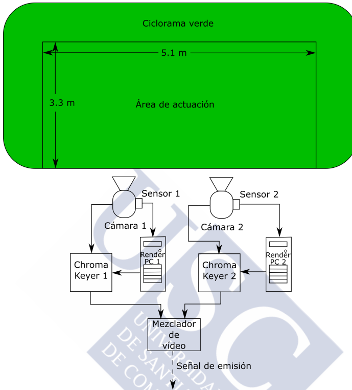
Figura 3.2: Esquema de conexiones del plató
