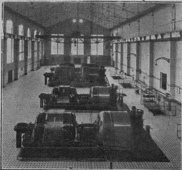
El nuevo salón de máquinas de Sorrento
