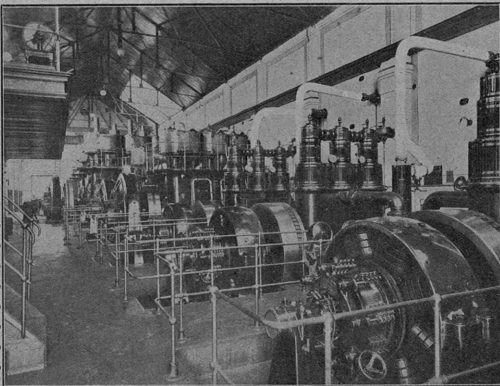
Sala de maquinarias de la usina
