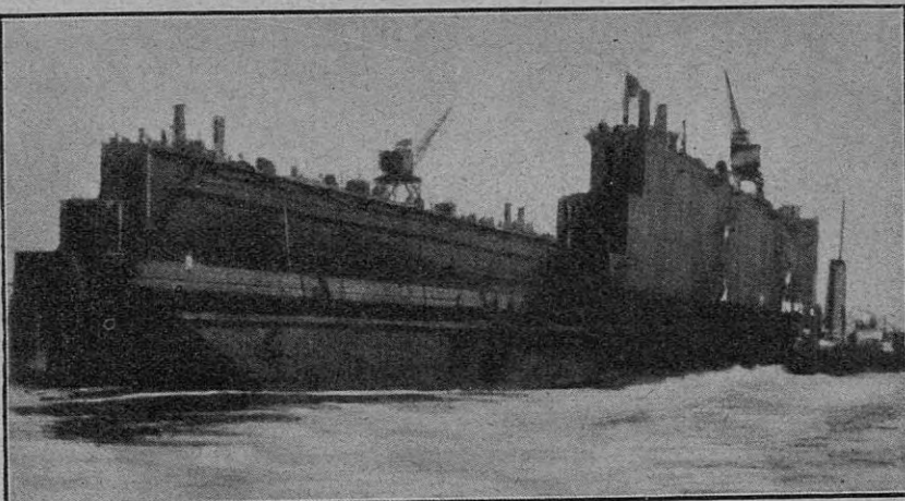
Nuevo dique de Portsmouth
