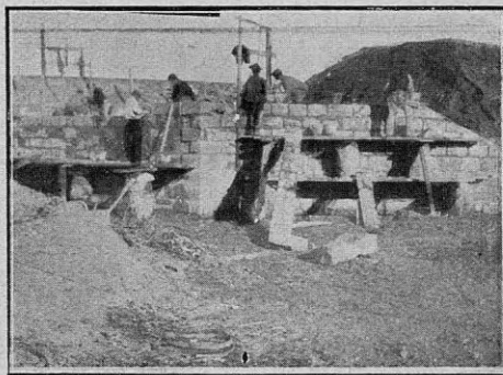
Puente sobre el Arroyo Seco, kilómetro 176. — Construcción de la mampostería de un estribo, con piedra labrada de la localidad
