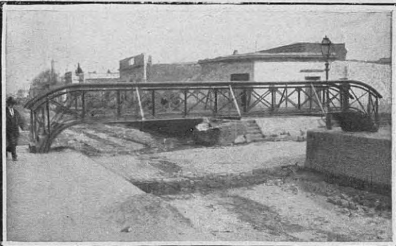
Tipo de los siete nuevos puentes que se colocarán sobre el zanjón Blanco Encalada, a la altura de las calles Arcos, Cuba, Obligado, Amenabar, Moldes, Vidal y Cramer
