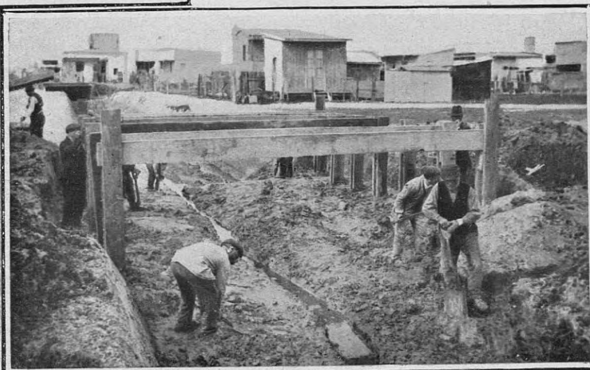
Ensanchando y rectificando el curso del caudaloso Teuco — calle del mismo nombre — y construyendo el puente de la calle Lynch
