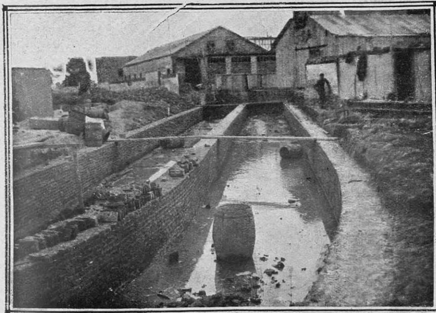
La parte del conducto de desagüe conocida por "La vuelta del Pobre Diablo" (Blanco Encalada y Migueletes), a punto de ser cubierta con tirantería de hierro y cemento armado, y sobre cuyo conjunto descansará el adoquinado
