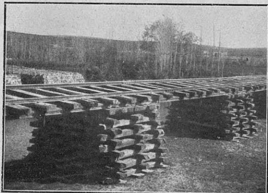
Puente provisorio sobre el arroyo Valcheta
