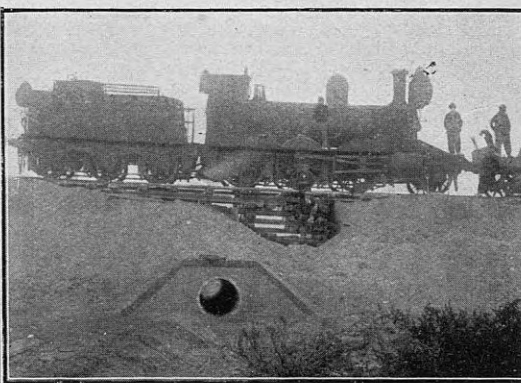
La máquina pasando por la alcantarilla definitiva, con restos de la provisoria
