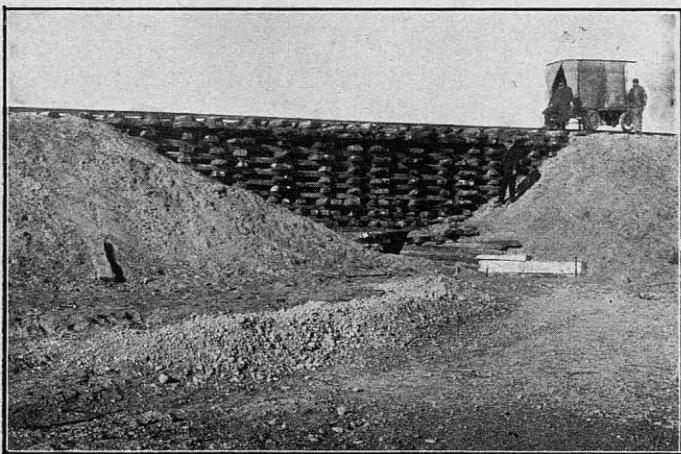
Una alcantarilla provisoria, hecha con durmientes
