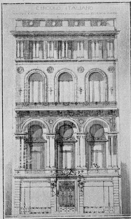
Frente del futuro edificio del Circolo Italiano, que será construido en la esquina de Florida y Corrientes, y sección transversal del mismo
