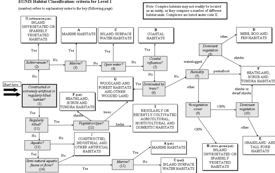
Figura 13.- Clasificación Eunis Hábitat. Clave principal de hábitats.
