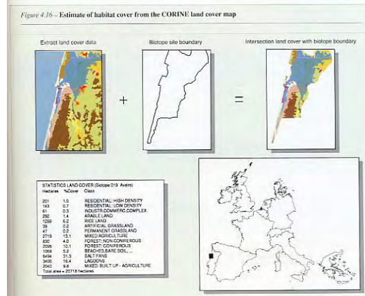
Figura 10.- Codificación de hábitats do proxecto CORINE Biotopos [esquerda]. Esquema de integración entre CORINE Biotopos e CORINE Land cover [dereita]
