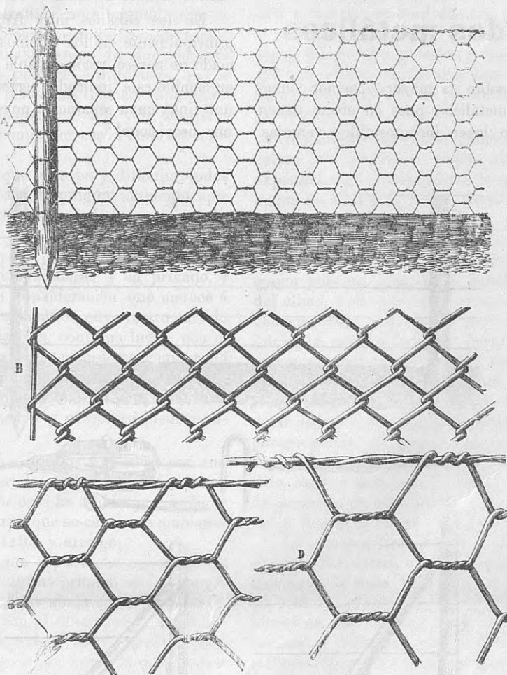
Figura 2. a Cercos con red metálica.— A Disposición de un cerco. B Red simple. C Red de mallas de doble torsión. D Red de mallas de cuatro torsiones.
