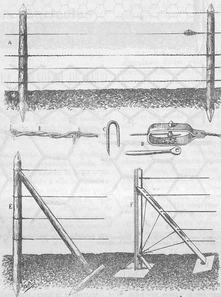
Figura 1.ª Cercas de hilo metálico. — A Cercado formado por dos hilos de alambre natural y tres de alambre armado. B Disposición de las puntas en el alambre armado. C Horquilla para clavar los alambres. D Torno y llave para tender el alambre. E Disposición de los postes en la extremidad de un cercado utilizando la madera. F La misma formada por barras de hierro.
